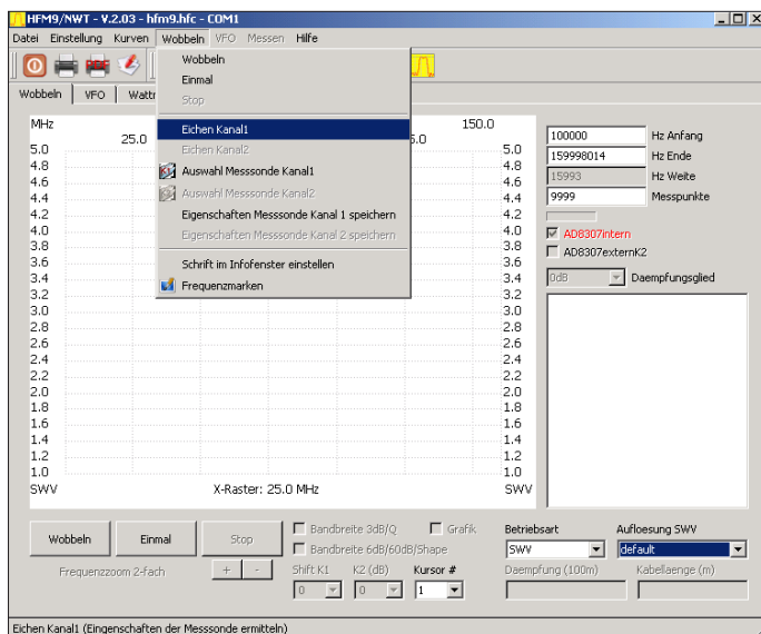
Bild 6: Der Reflexionsmesskopf muss auch in der aktuellen Softwareversion WinNWT 2.03 von DL4JAL nach dem ersten Anstecken kalibriert werden – dazu ist Arbeitsblatt Wobbeln , Betriebsart SWV , im Menü Wobbeln der Unterpunkt Eichen Kanal 1 zu wählen; Abspeicherung am besten unter defsonde1 .
