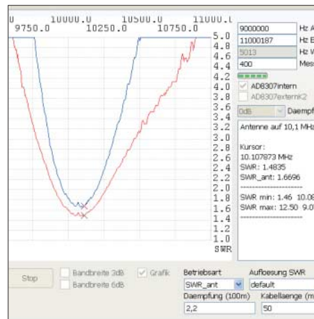
Bild 11: SWV-Verlauf der Multiband-Antenne aus Bild 9 im 30-m-Band, gemessen mit WinNWT; in der Betriebsart SWR_ant erfolgt nach Eingabe der 100-m-Dämpfung und der tatsächlichen Länge des Kabels eine Rückrechnung auf das SWV an der Antenne (rote Kurve).
